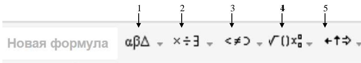
Рисунок 12. Панель формул.
