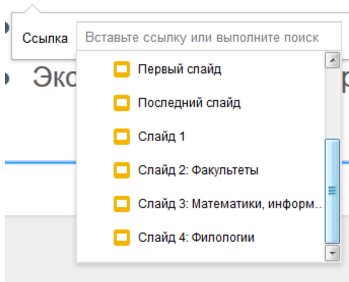
Рисунок 21. Создание гиперссылки.
